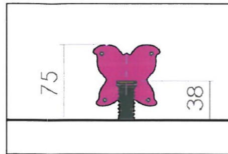
Клатушка "Пеперуда" Изглед-габарити
