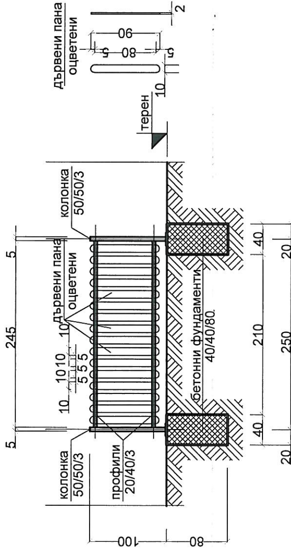
ОГРАДНО ПАНО M1:50
