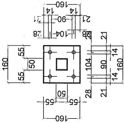
ДЕТАЙЛ ОСНОВНА ПЛОЧА 160/160/8 M1:50
